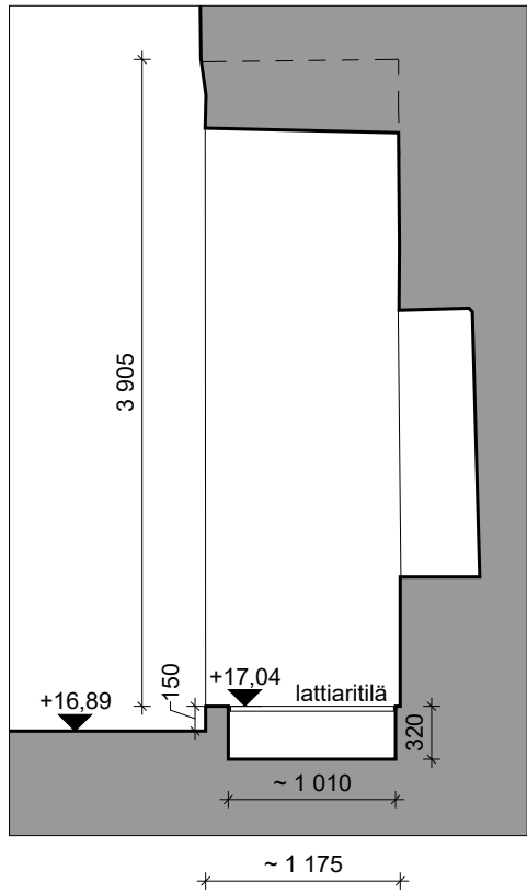
Leikkaus 1 1:50
